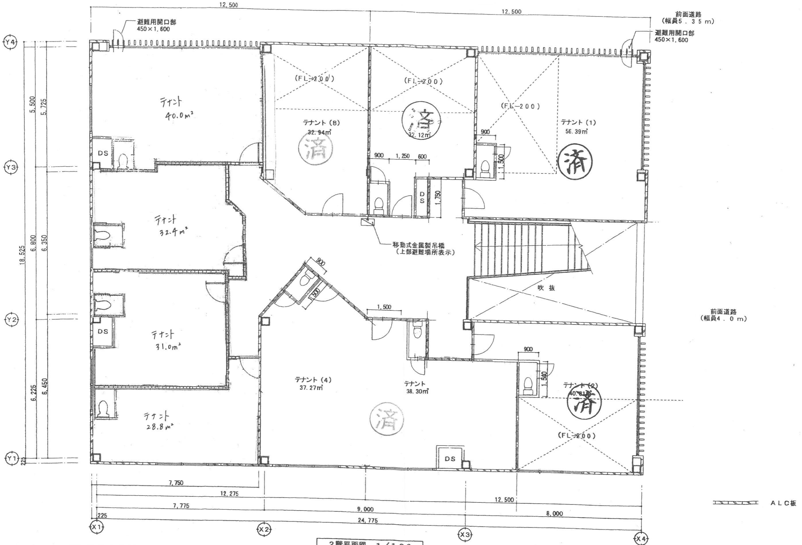
2階平面図 1/100
